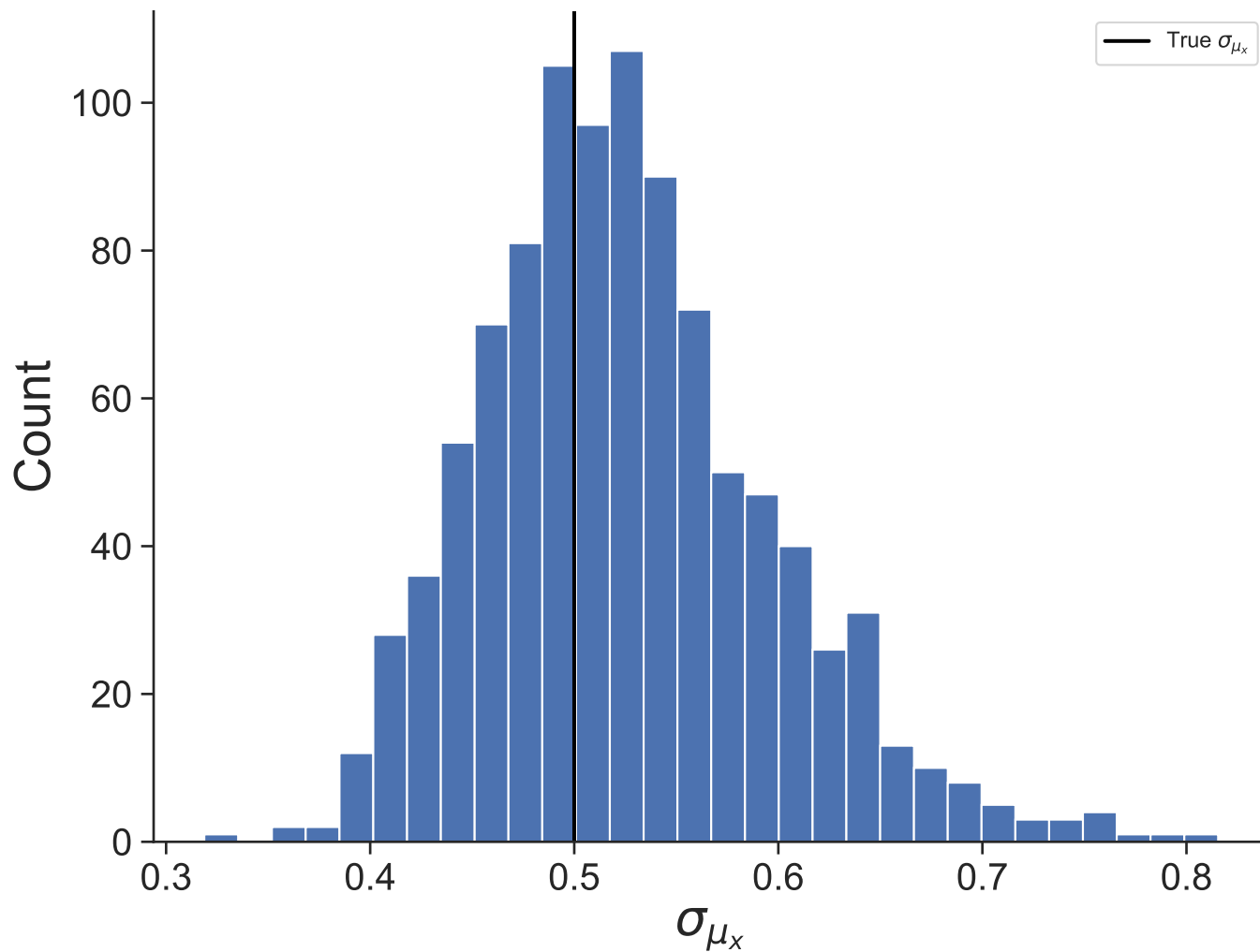
Dataset 45
