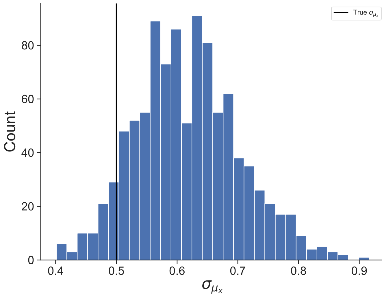
Dataset 38
