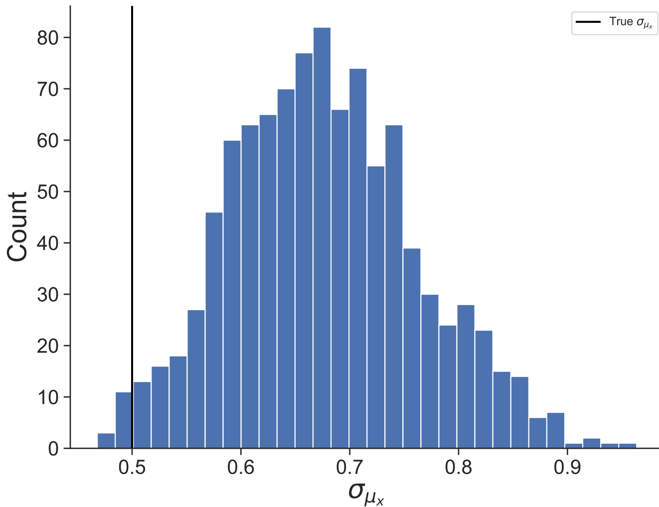
Dataset 20
