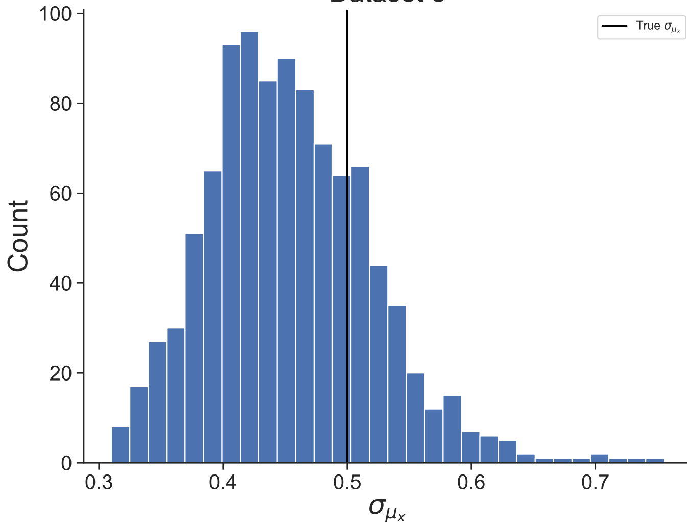
Dataset 8
