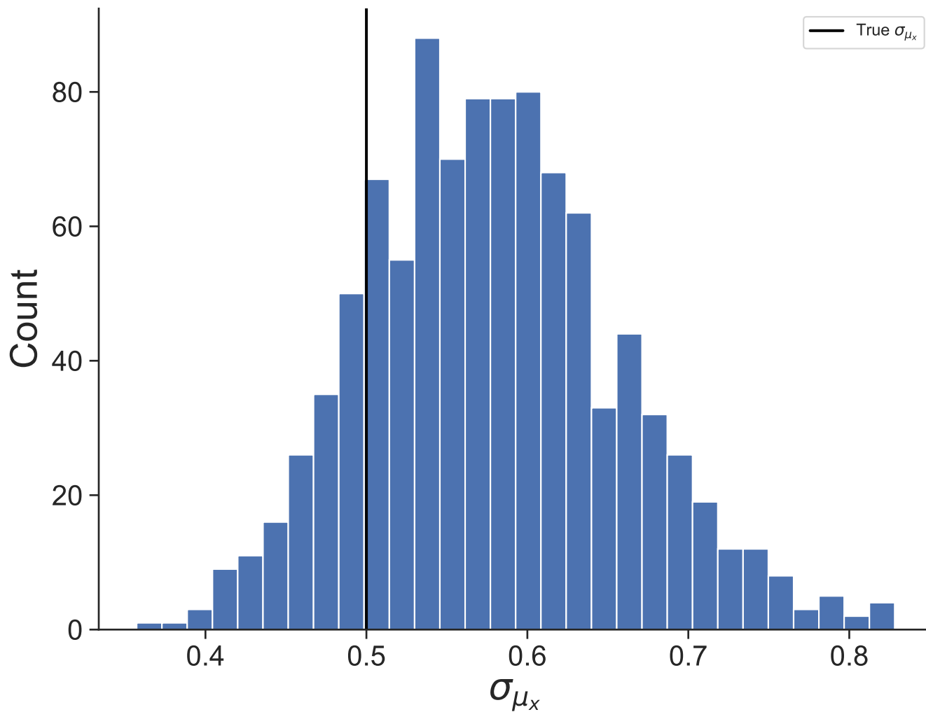
Dataset 3
