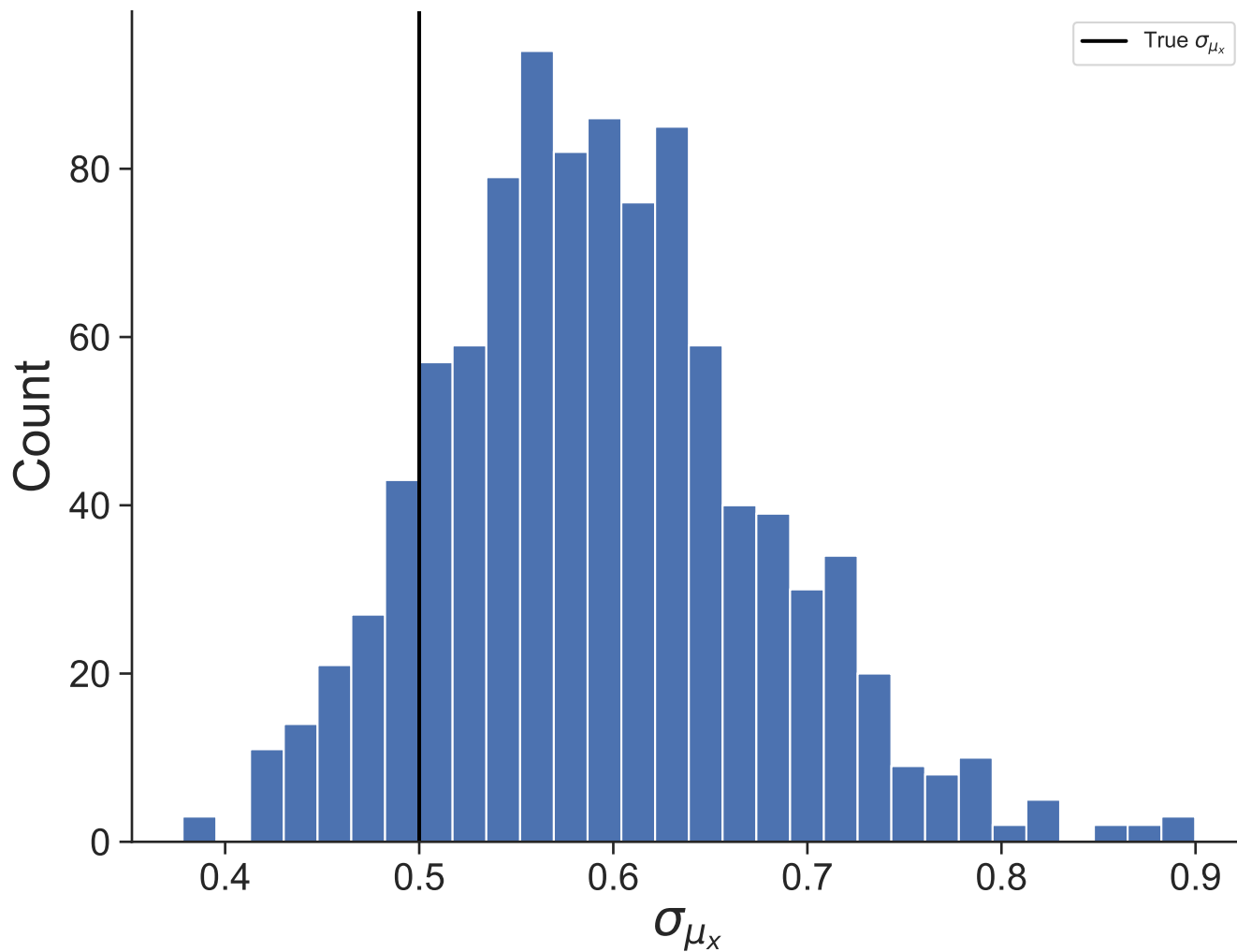
Dataset 43
