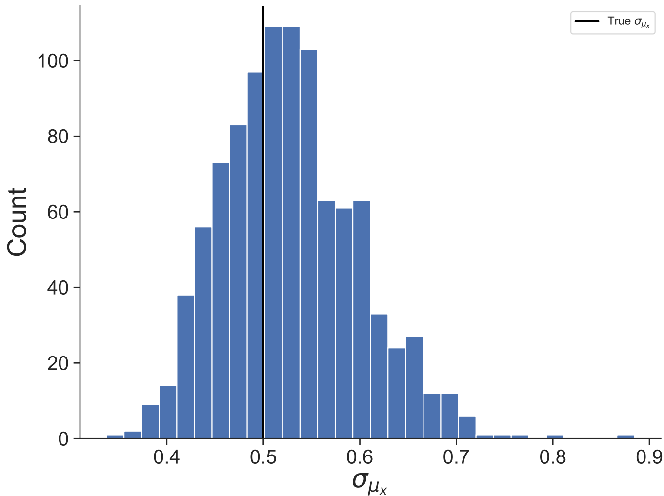
Dataset 32
