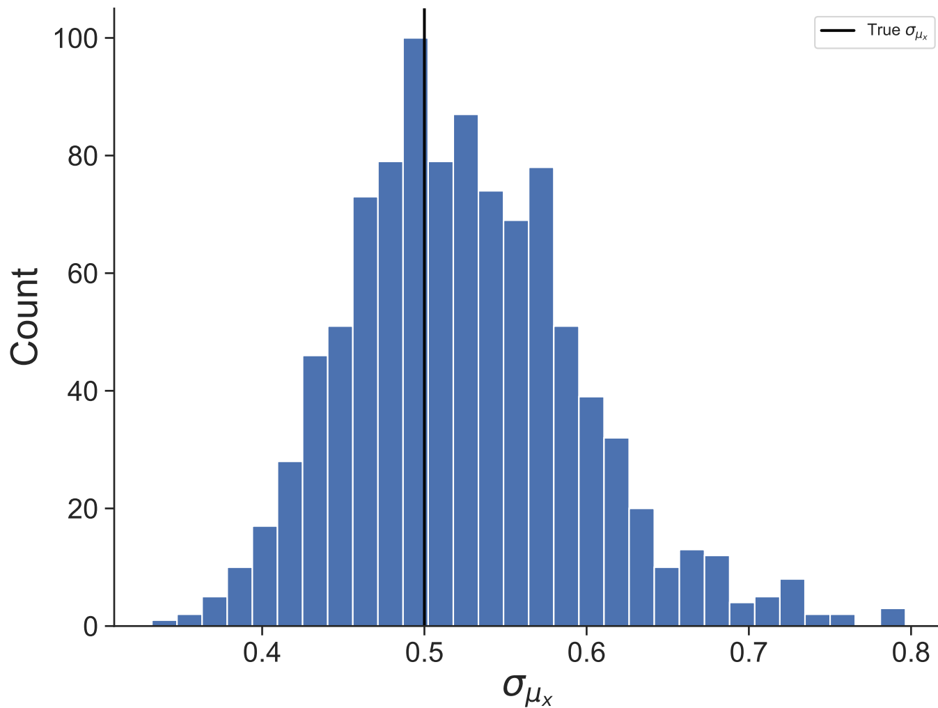
Dataset 46
