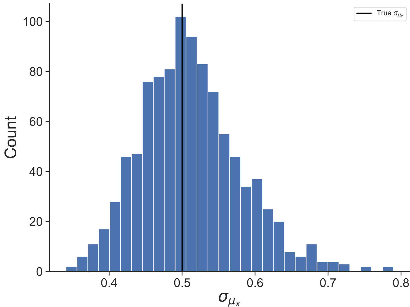
Dataset 17
