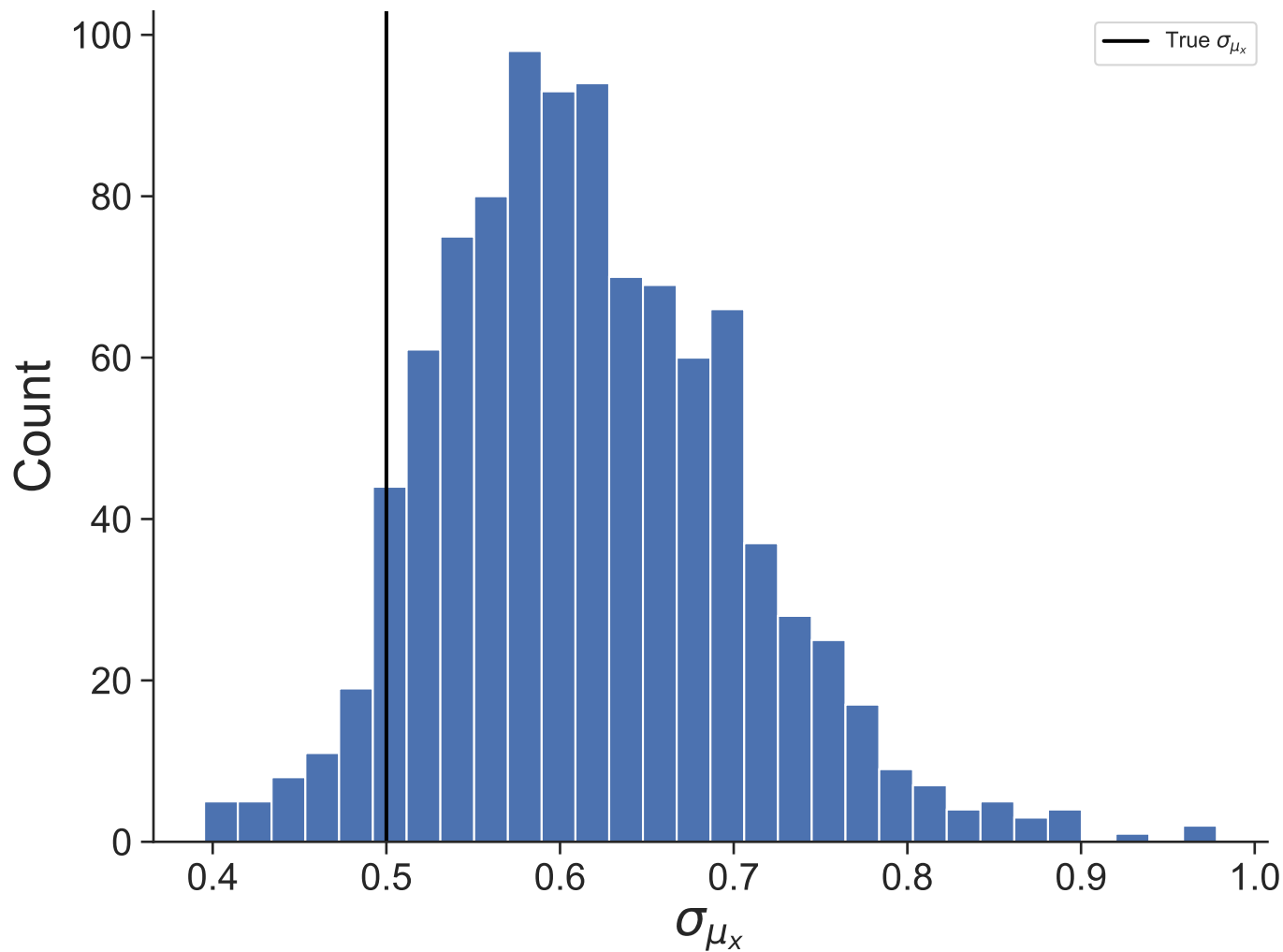
Dataset 15
