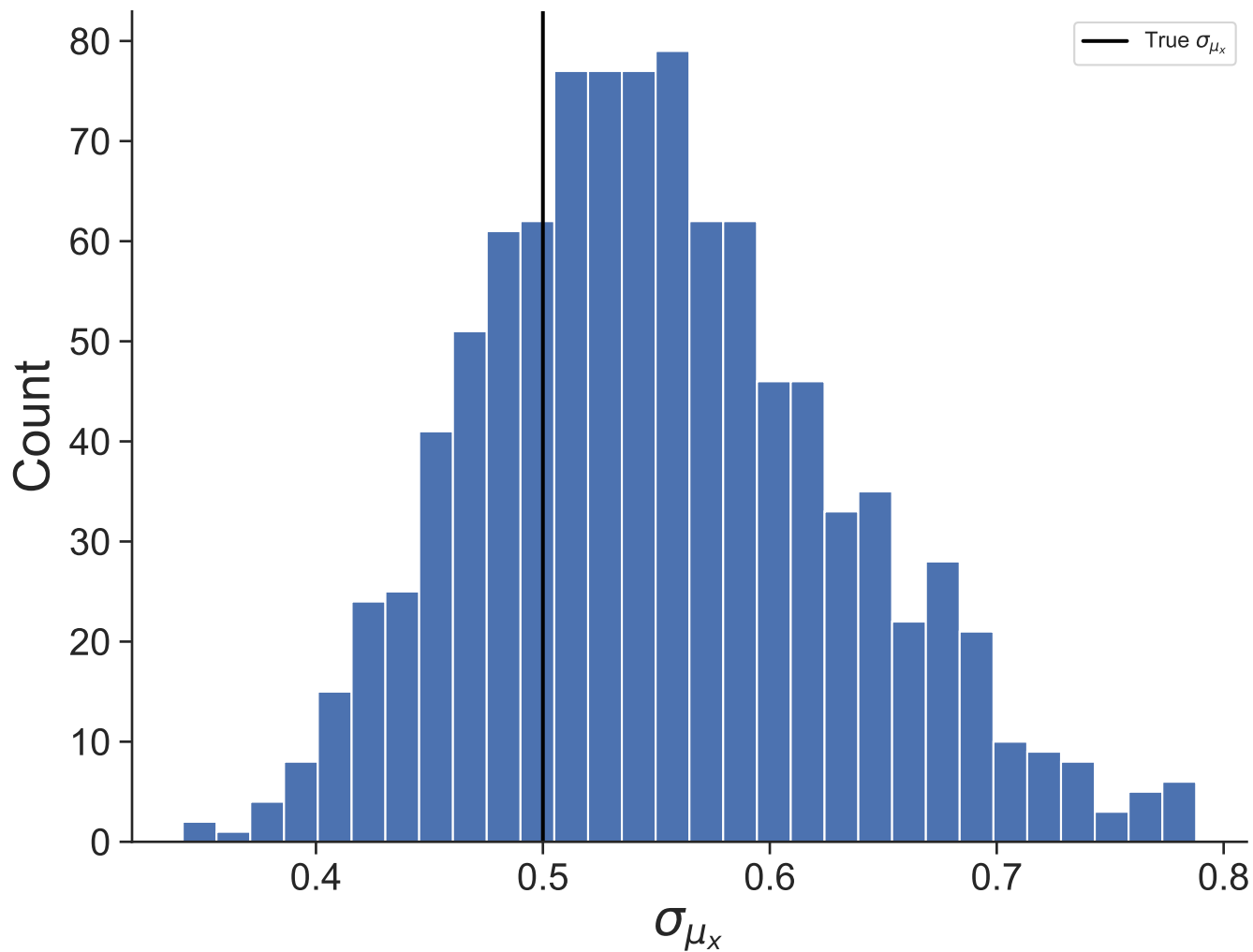
Dataset 41
