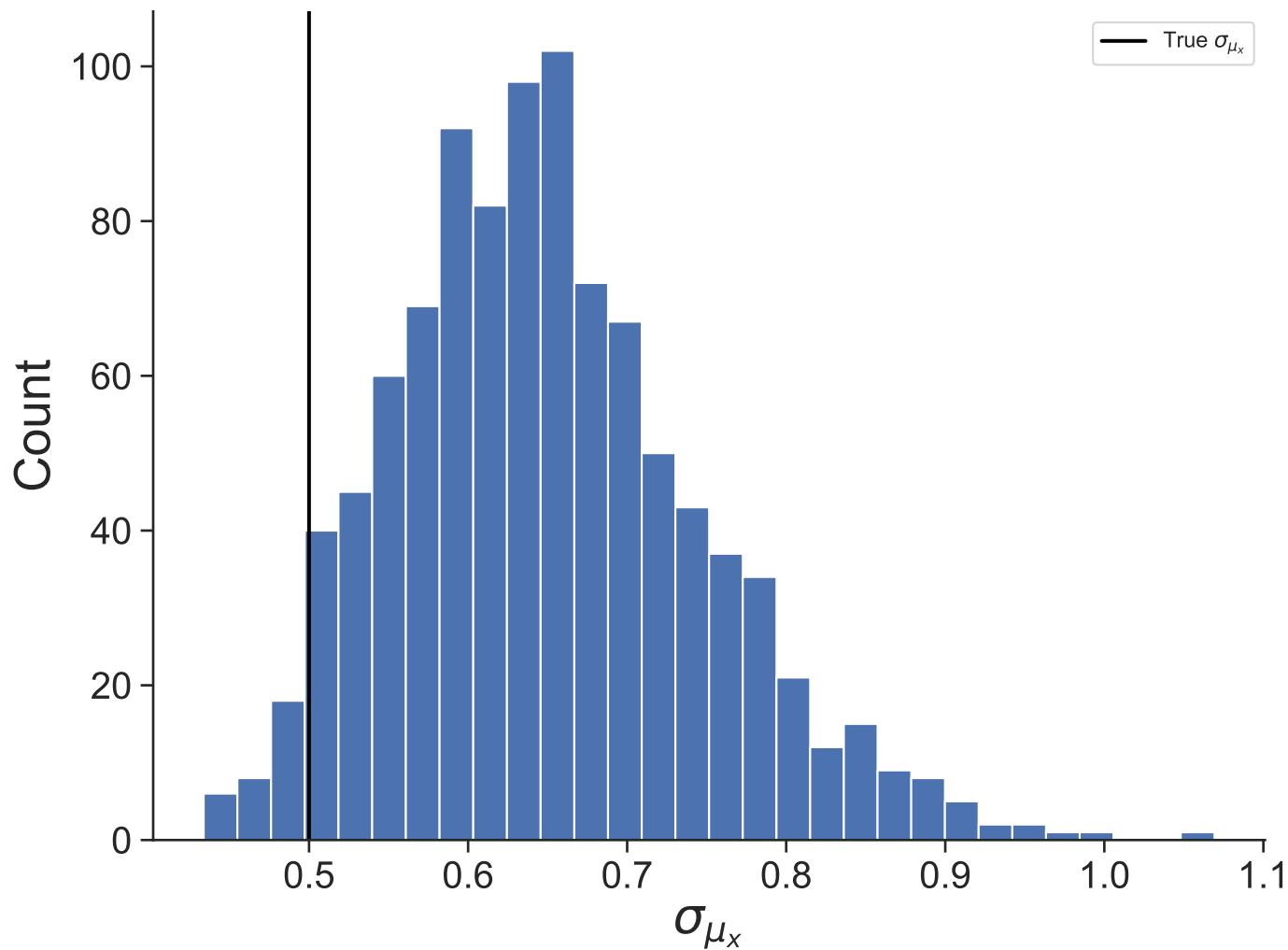
Dataset 6
