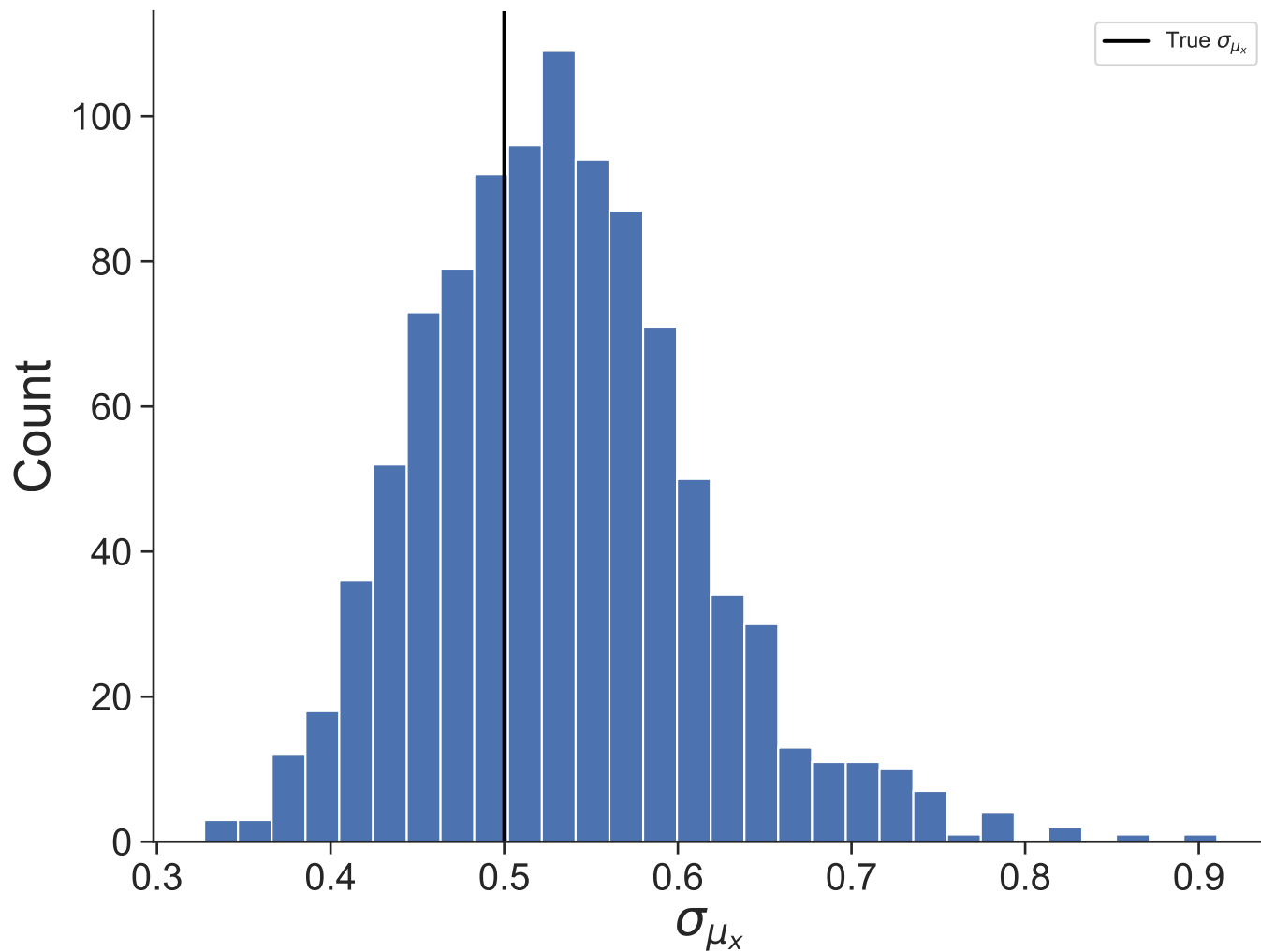
Dataset 40
