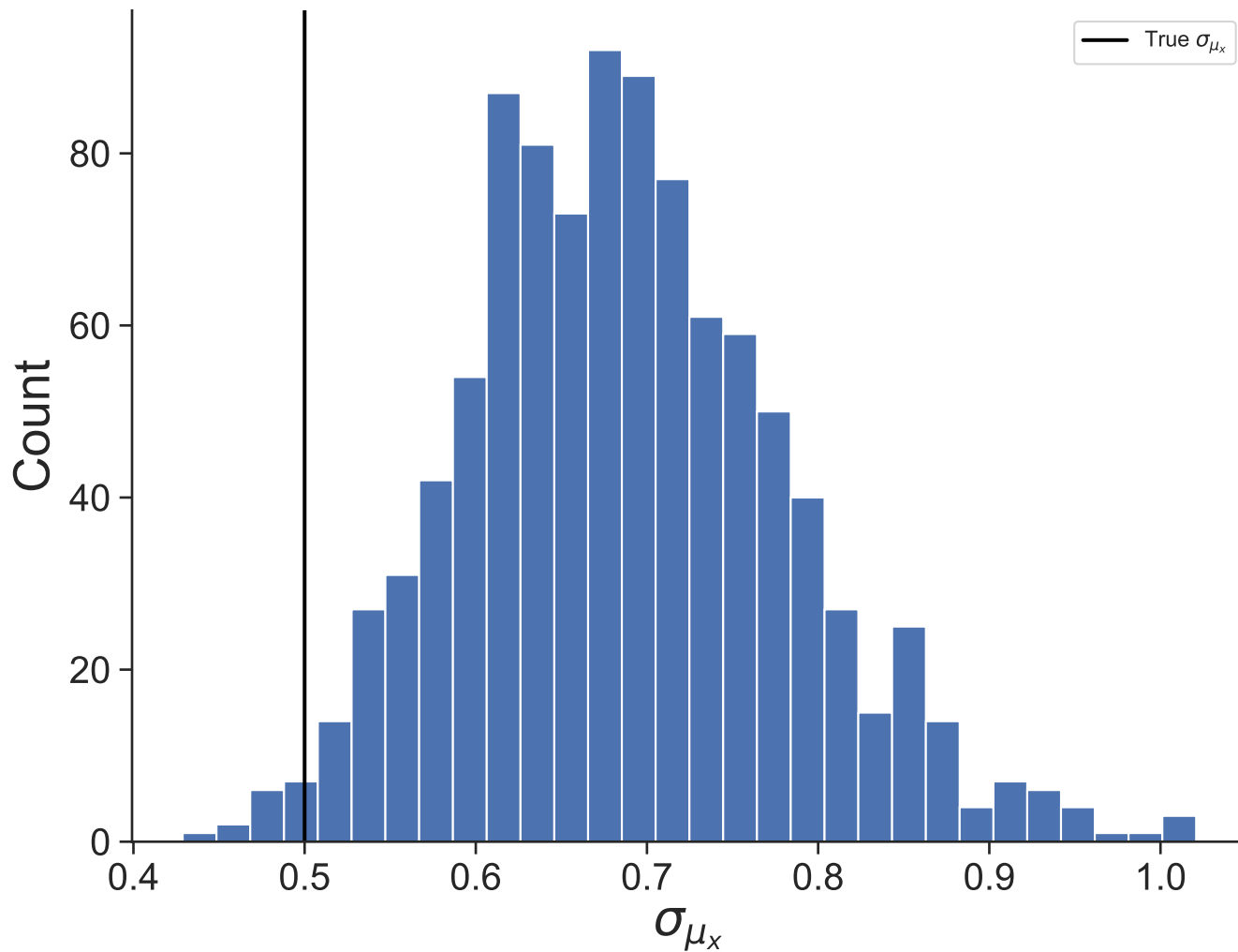
Dataset 16
