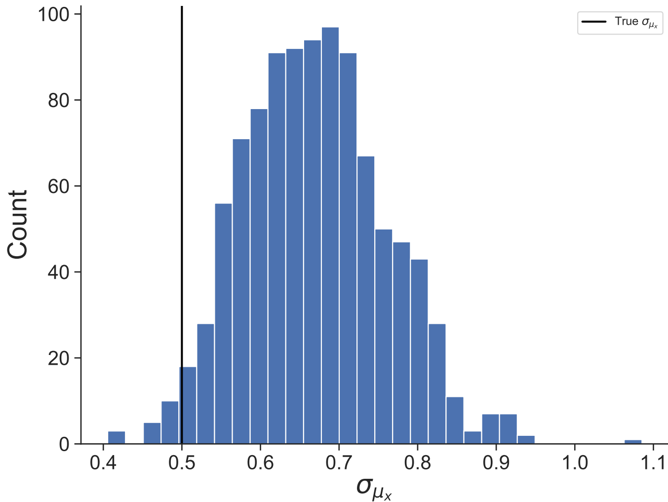
Dataset 24
