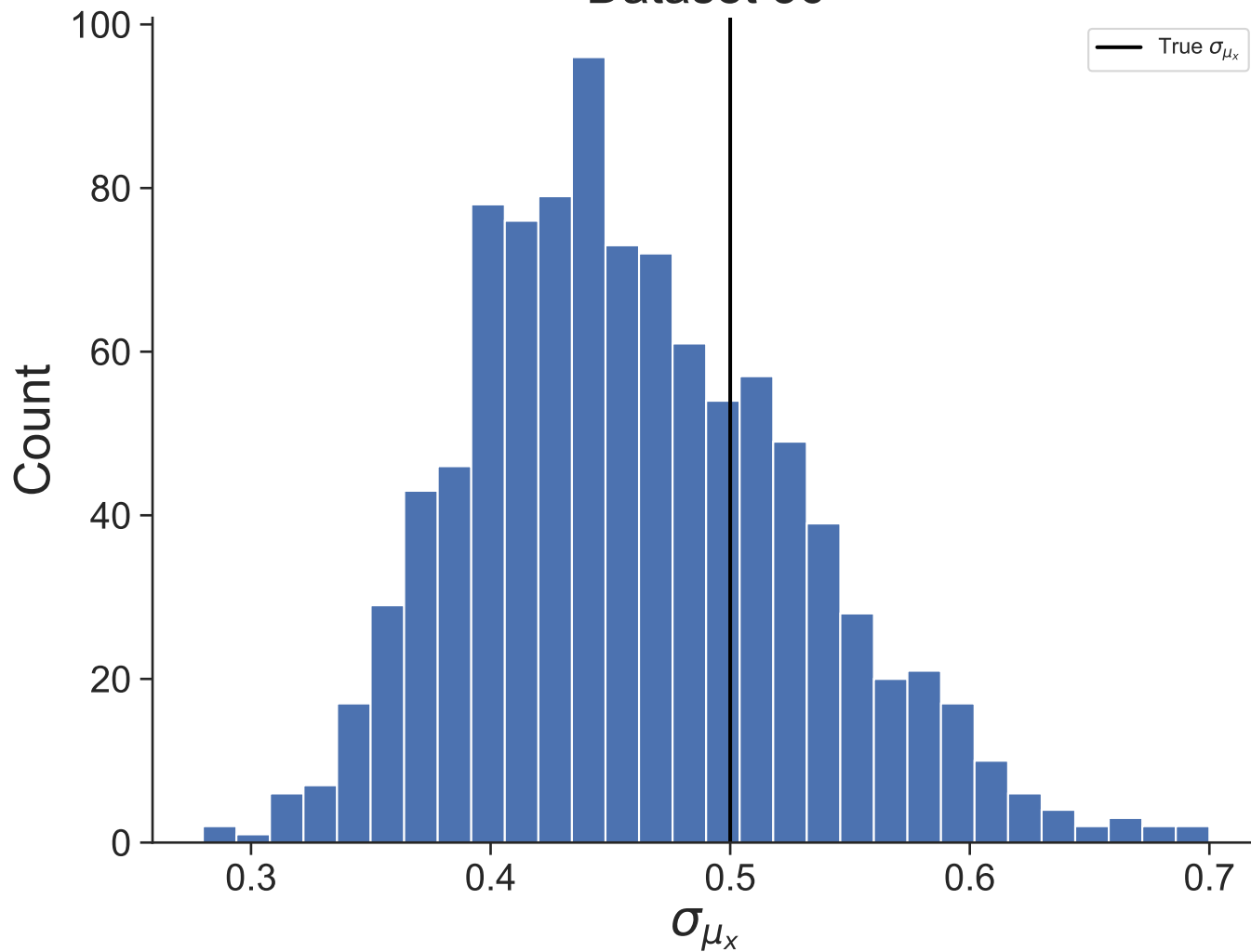
Dataset 36
