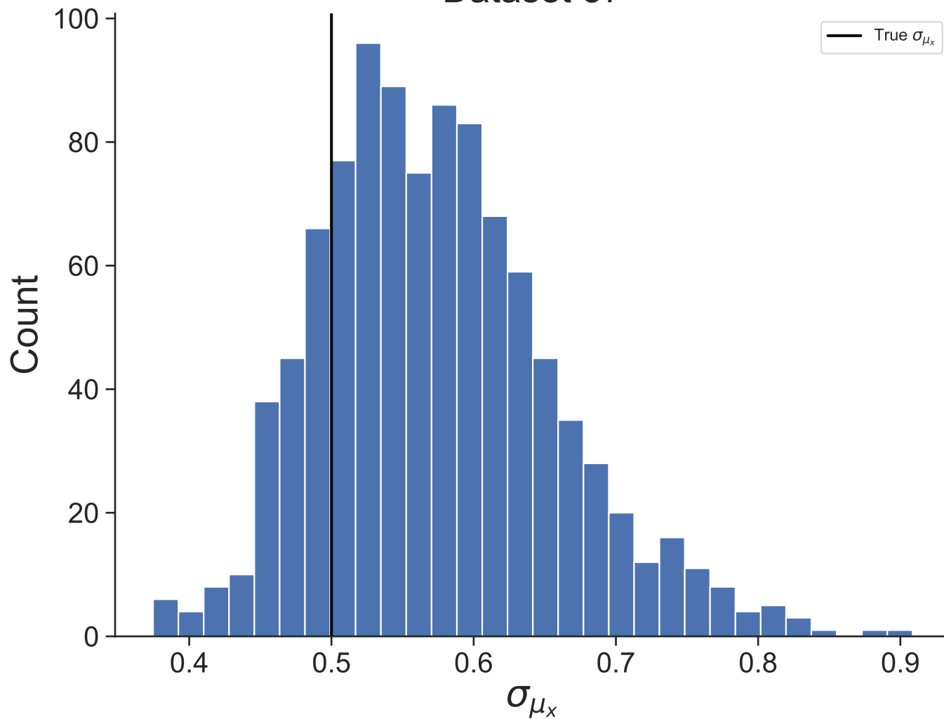
Dataset 37
