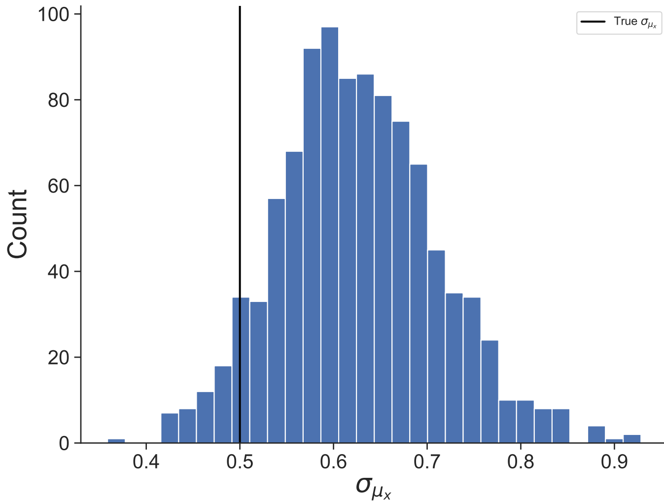
Dataset 19
