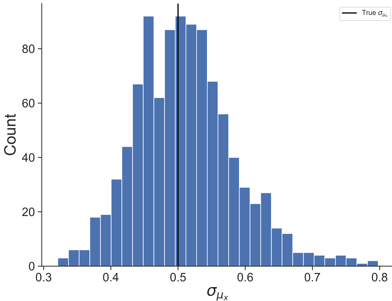
Dataset 9
