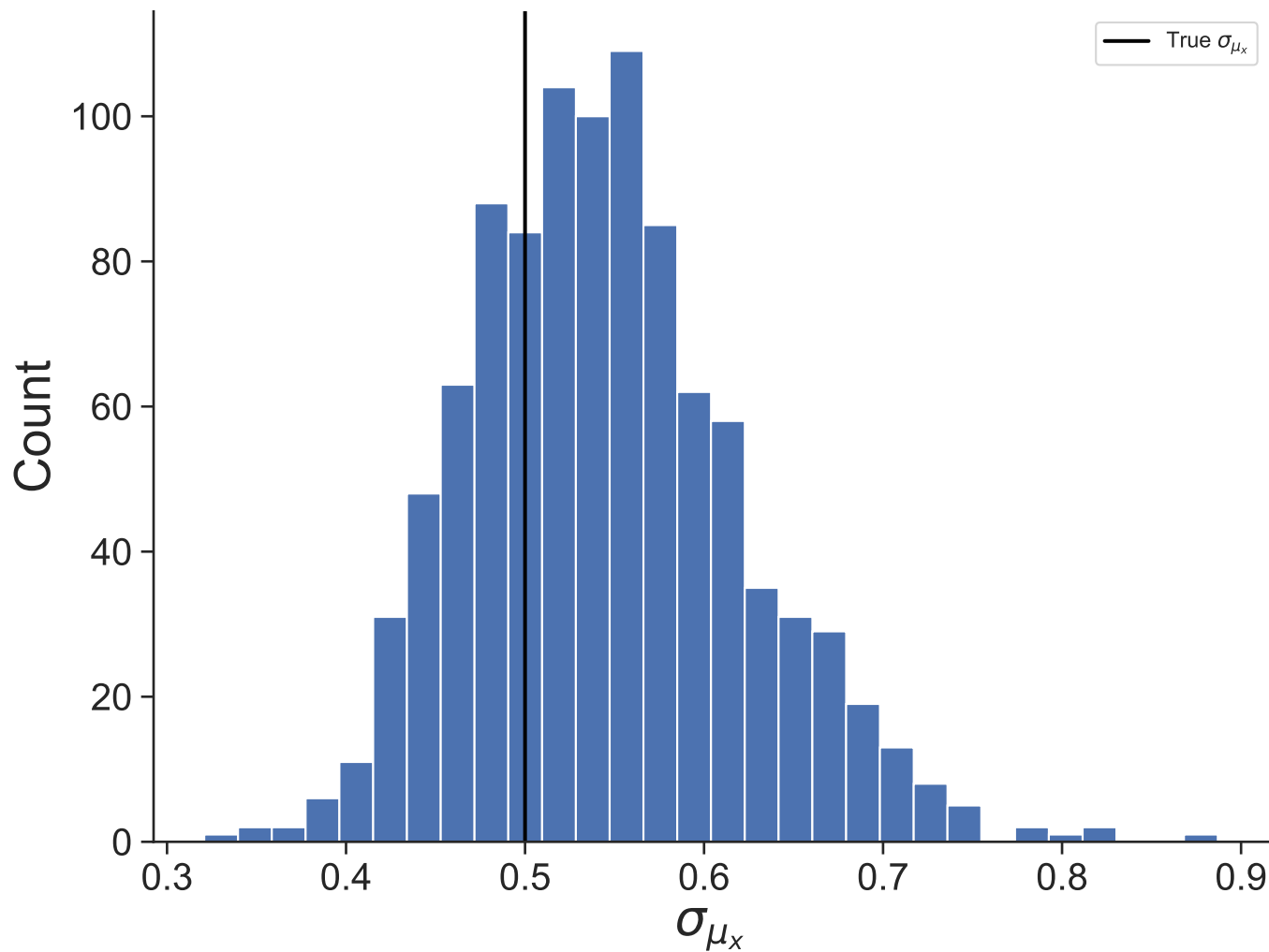
Dataset 29
