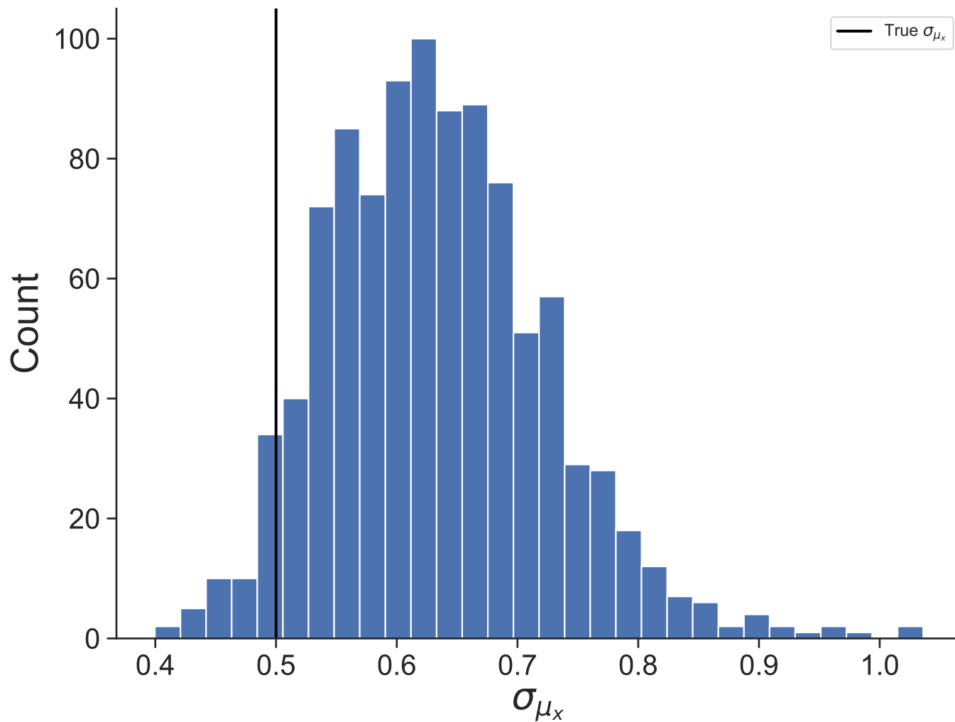
Dataset 22
