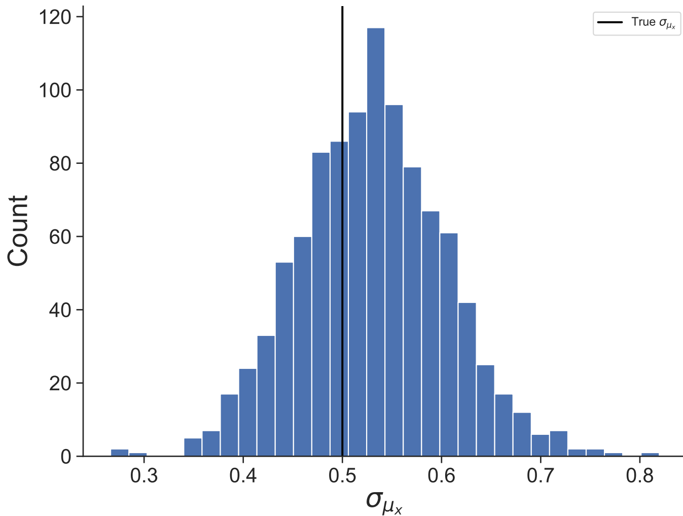
Dataset 33
