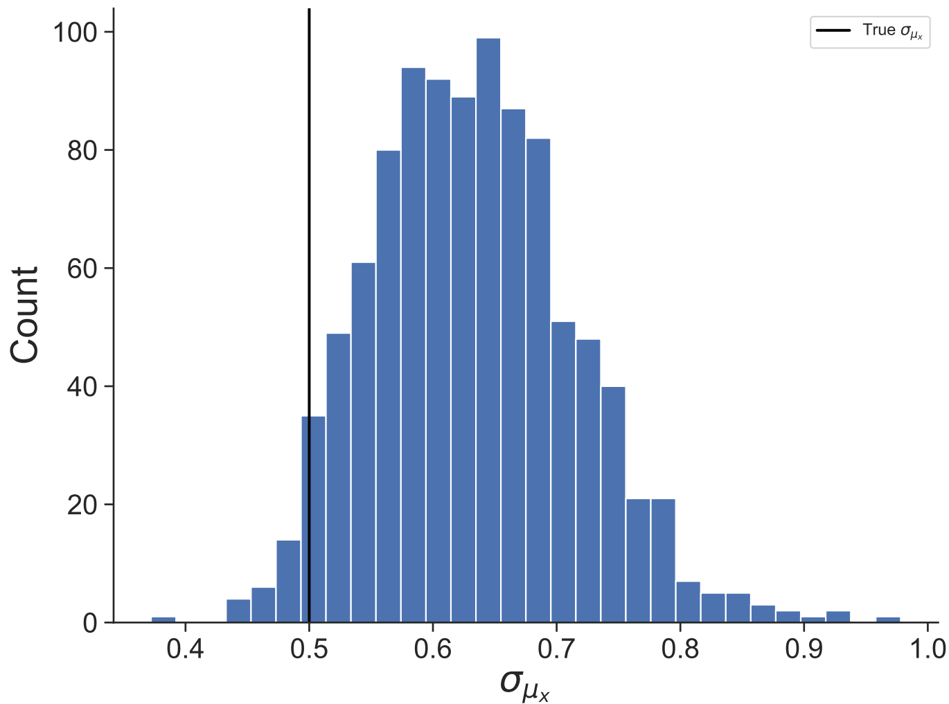
Dataset 42
